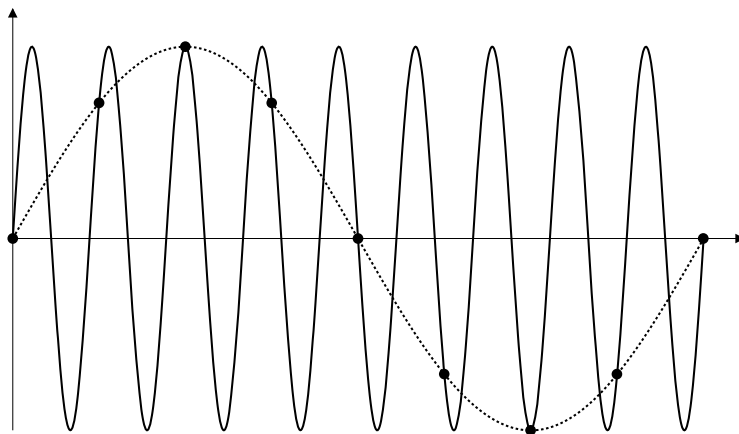
Рис. 21 Наложение спектров
