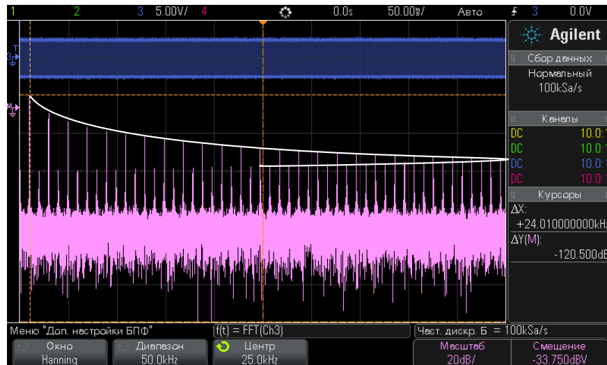
Рис. 7 Наложение спектров
